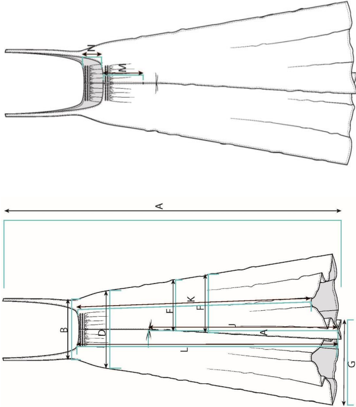
Technische Zeichnung
